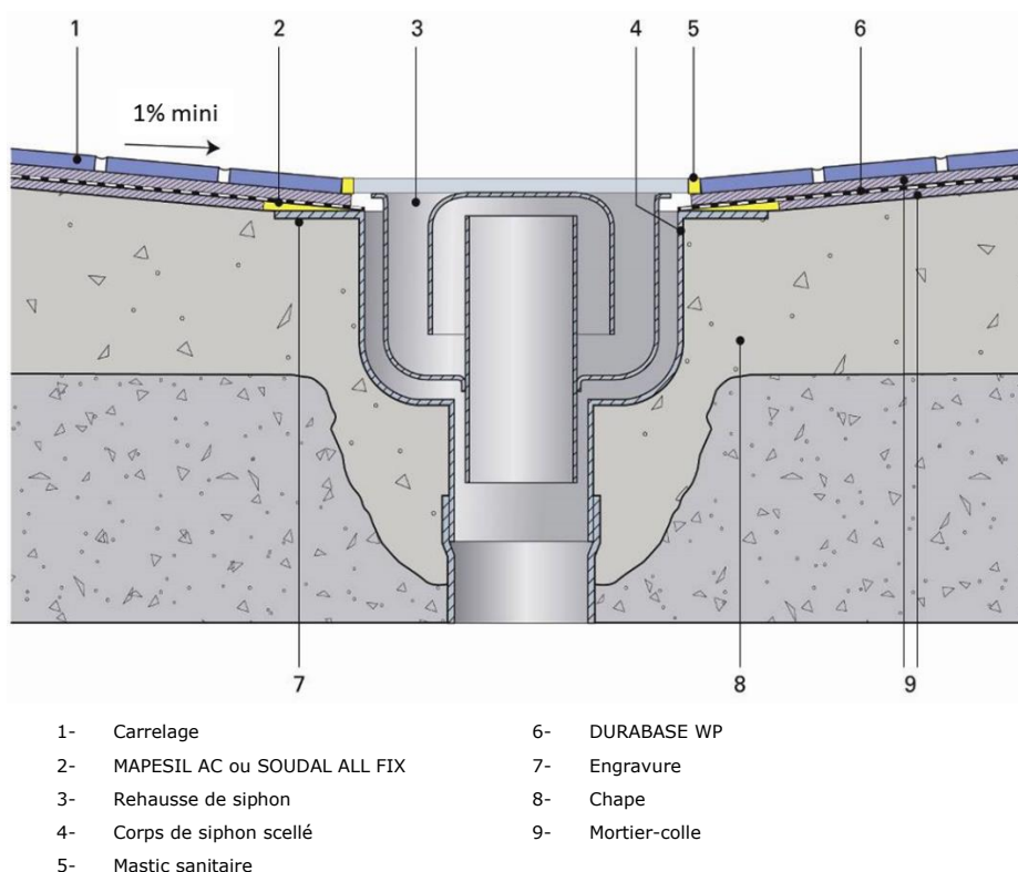
Figure 4 - Siphon de sol en pose collée
