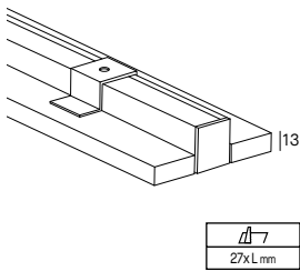
KIT/TRIM/PA12 Kit incasso trimless per PA/12 (2pz)
