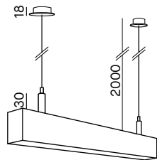
KIT/SOSP/PA Kit sospensione per PA/12 (2pz)
