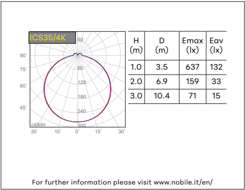
SQUARE LUMINAIRE
